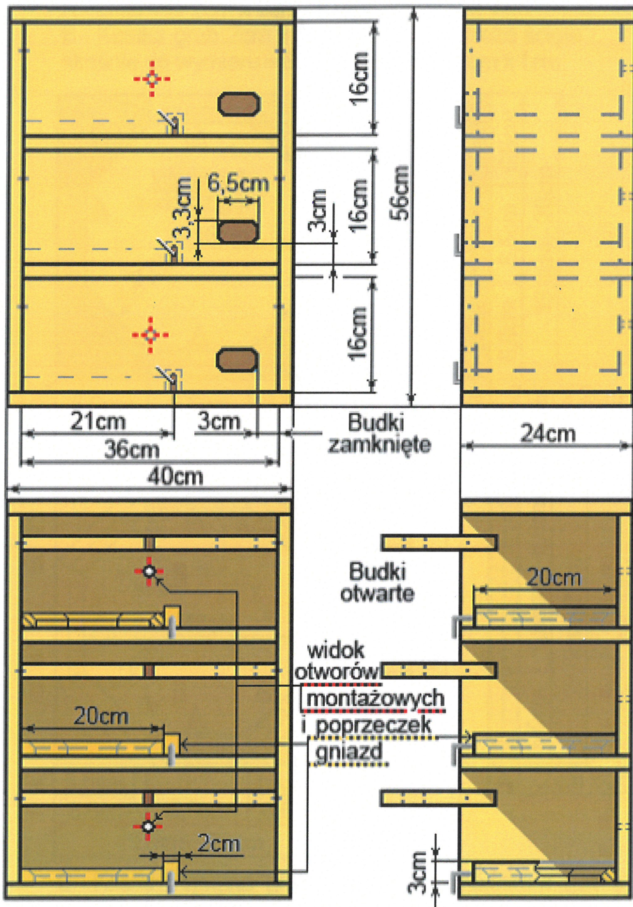
Załącznik projektu Budżetu Obywatelskiego 2023: Budki dla jerzyków na placówkach publicznych Segment 3-budkowy
